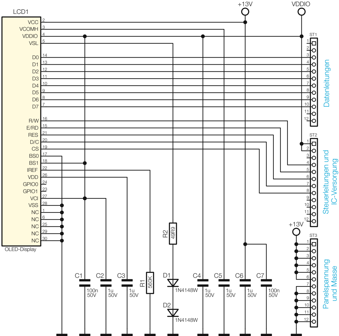
Bild 8: Die Schaltung des OLED-Moduls
