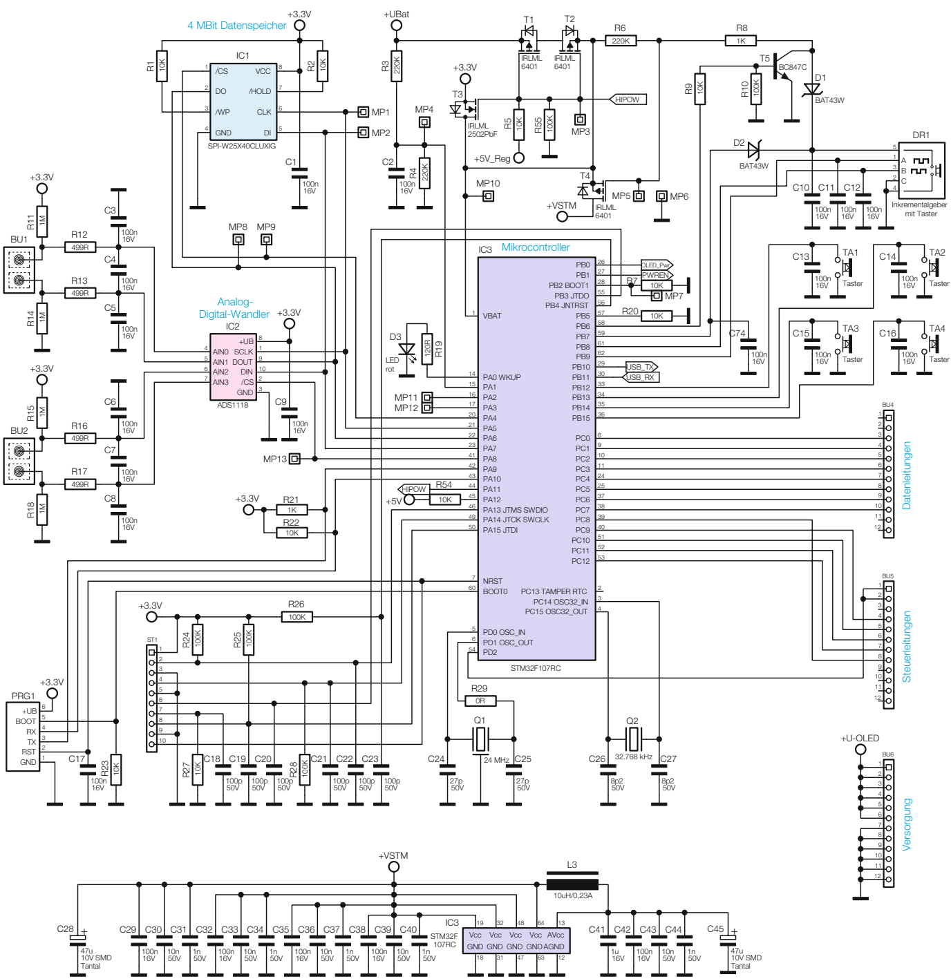
Bild 6: Das Schaltbild des TD0200 mit Mikrocontroller, ADC, Datenspeicher, Bedien- und Anzeigeelementen
