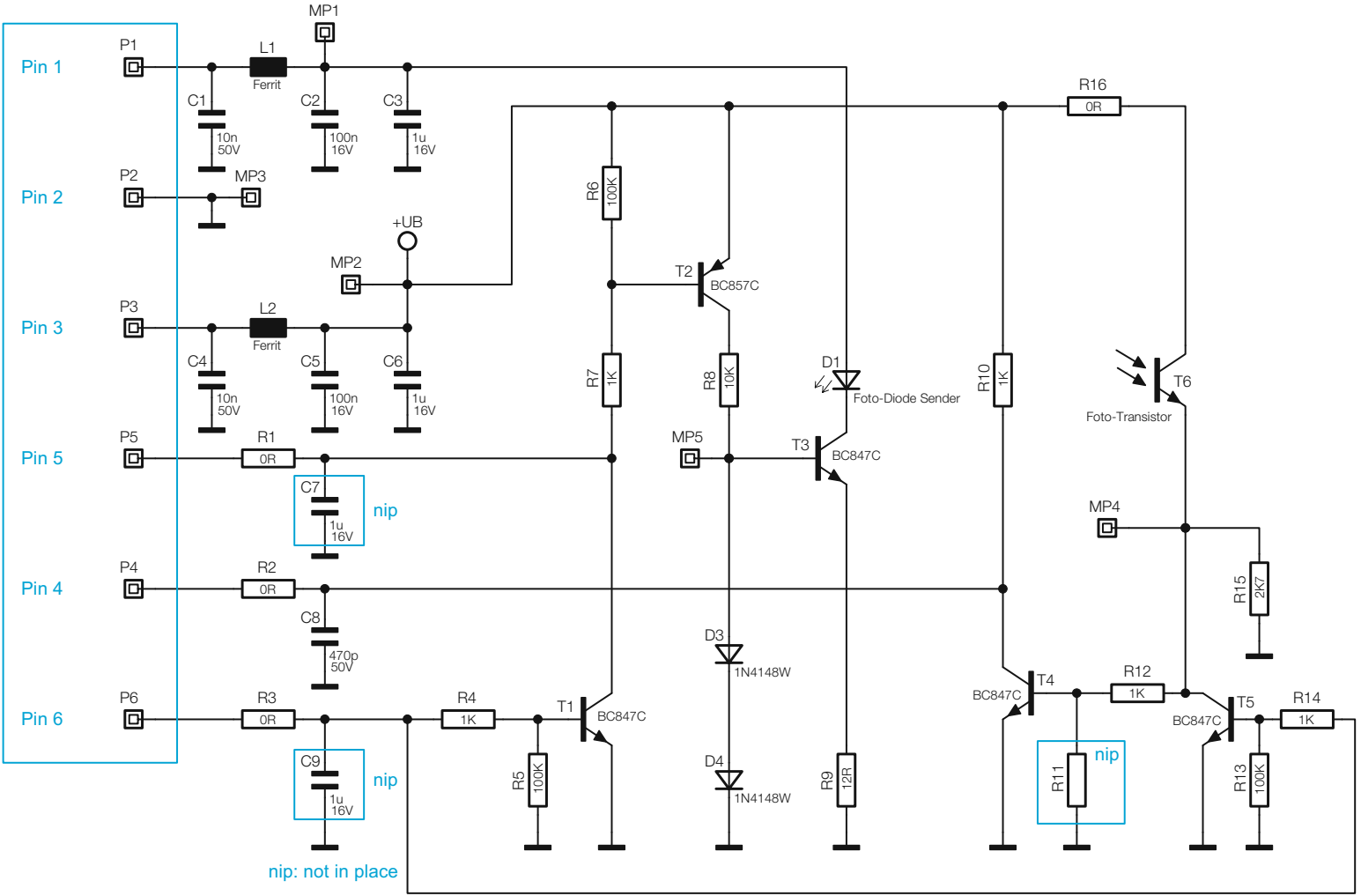
Bild 4: Das Schaltbild des Energie-Sensors ES-IEC
