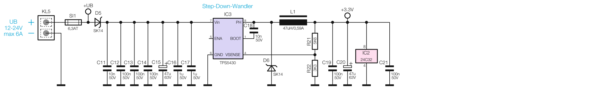
Bild 7: Das Schaltbild des HomeMatic-RGBW-Controllers
