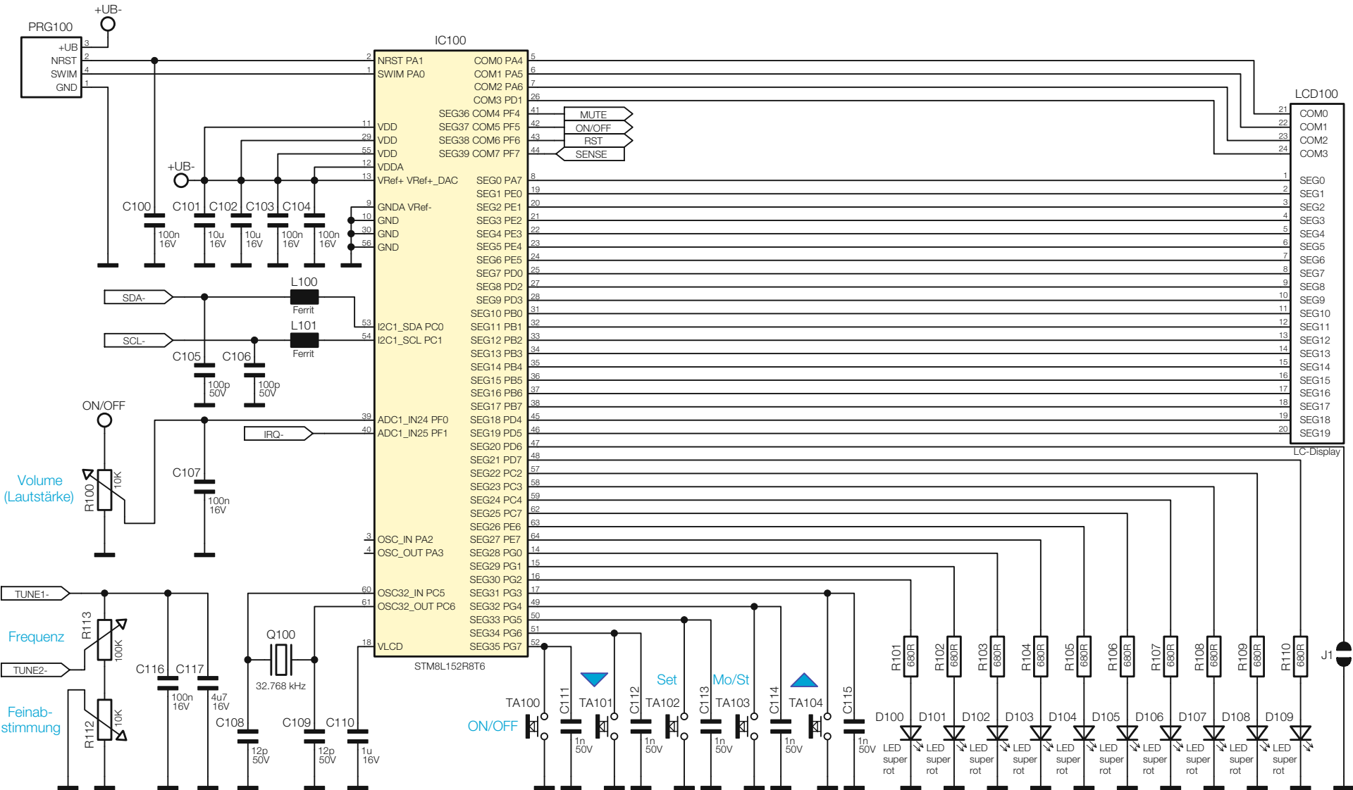
Bild 4: Schaltbild des Controller- und Bedienteils, der sich auf der Bedienplatte befindet
