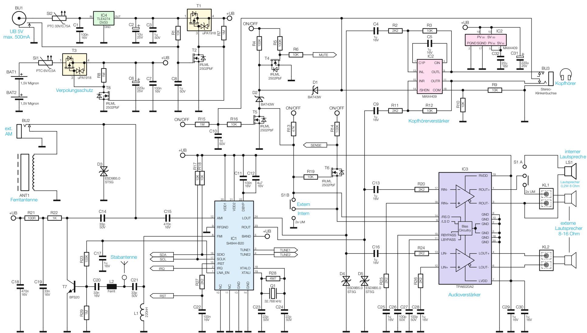
Bild 3: Schaltbild des Empfängerteils, der sich auf der Hauptplatine befindet
