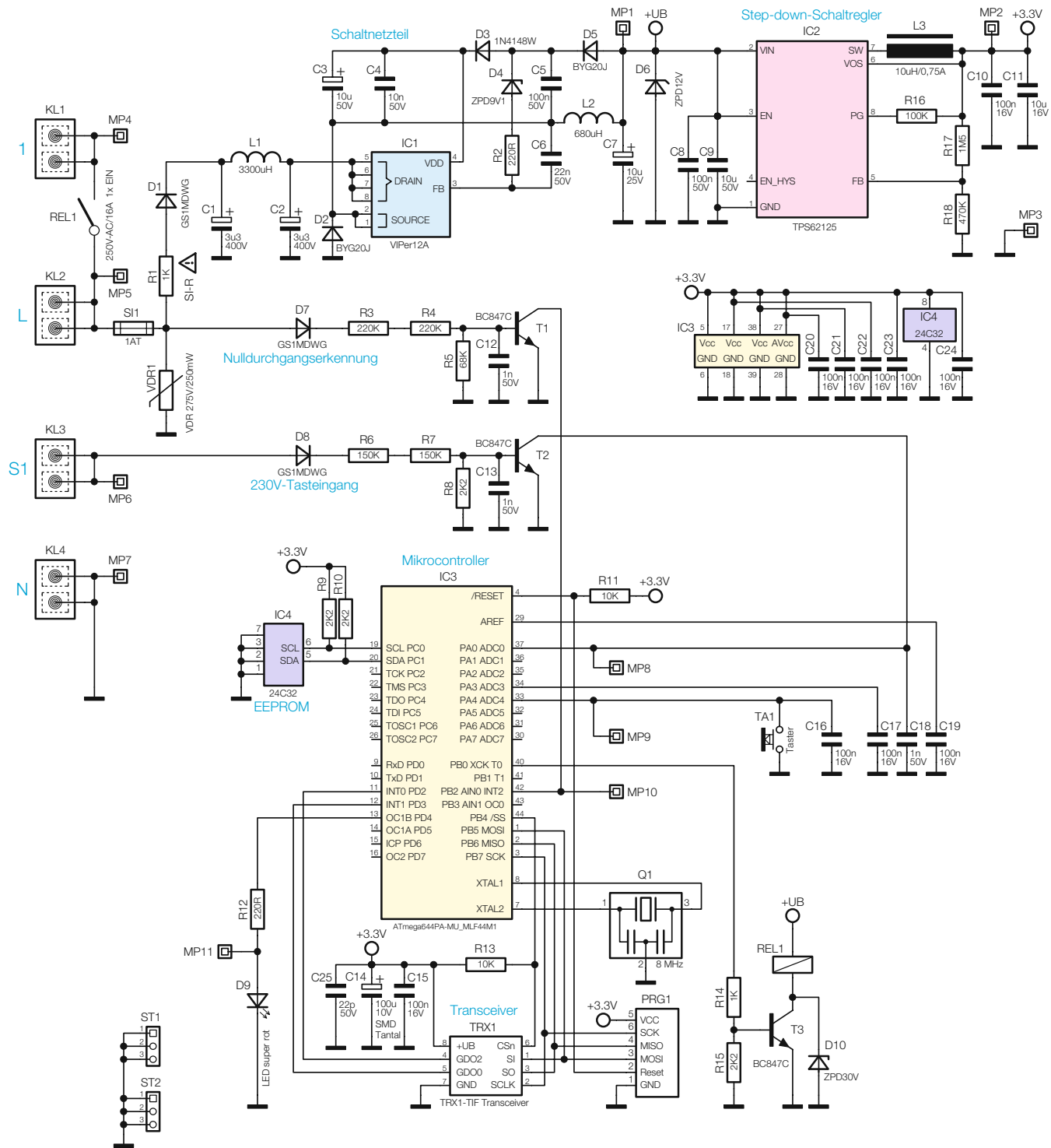
Bild 1: Das Schaltbild des Schaltaktors
