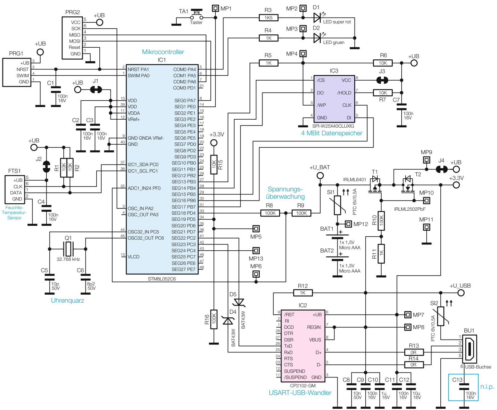
Bild 1: Das Schaltbild des TFD 500
