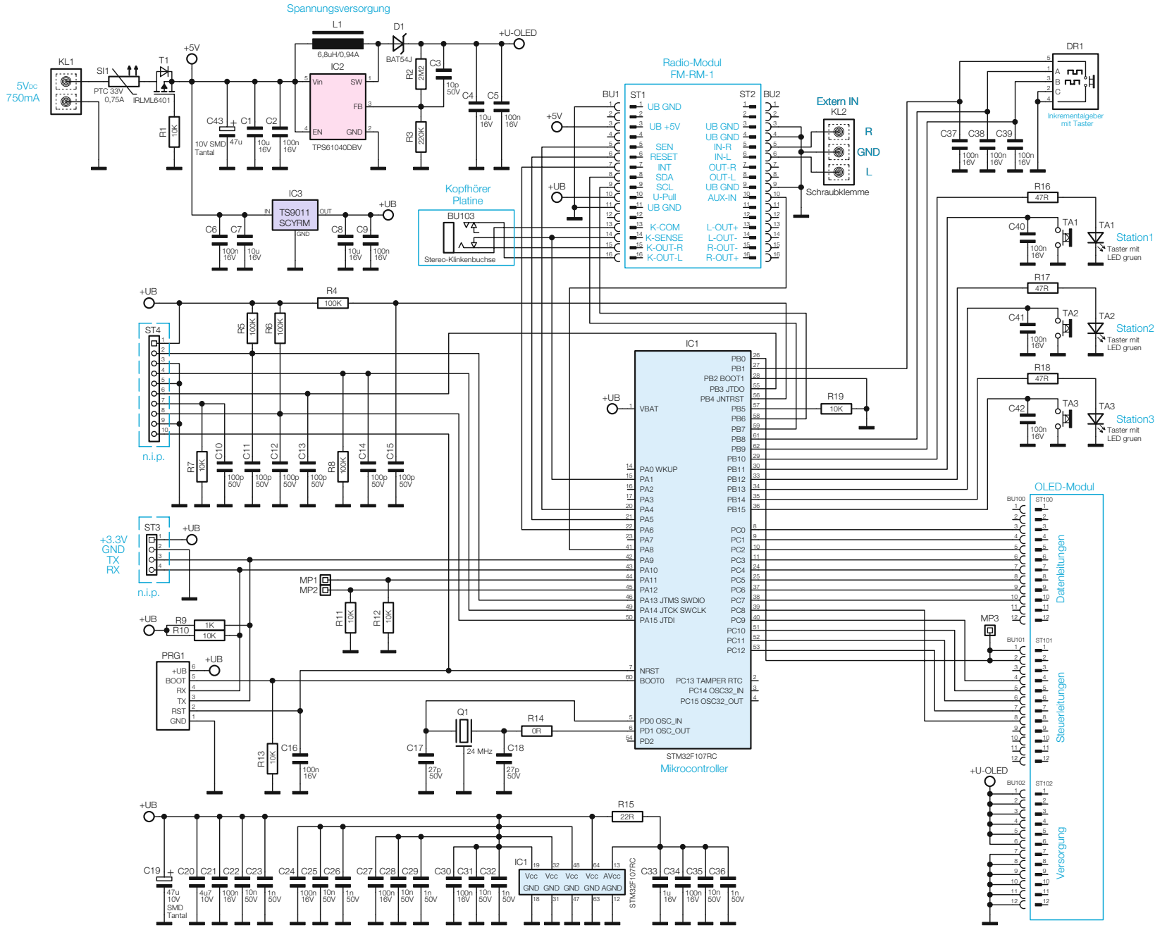
Bild 5: Das Schaltbild der Bedien- und Anzeigeeinheit für das FM-RM1
