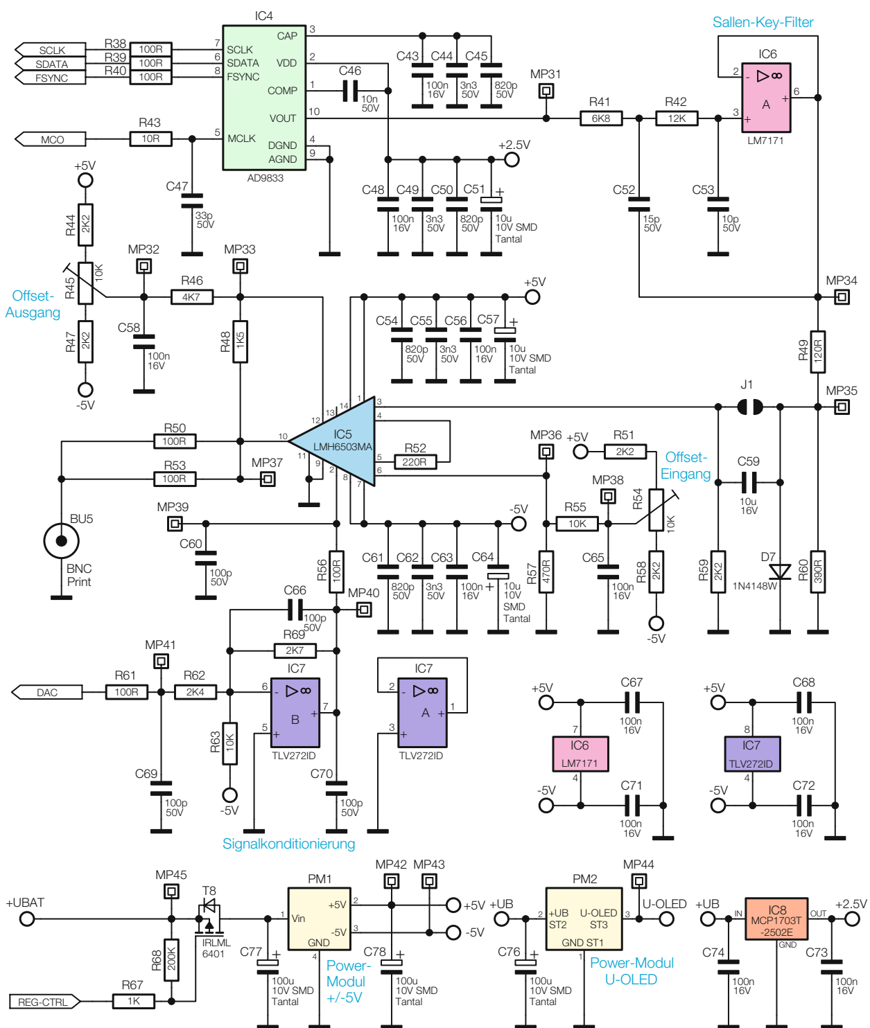
Bild 3: Schaltbild der Signalerzeugung per DDS-Chip und des Verstärkteils
