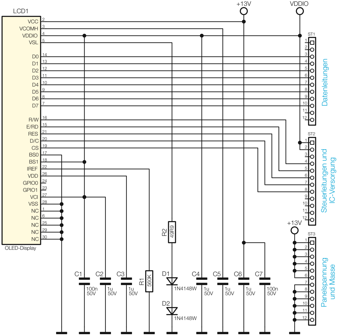
Bild 4: Schaltbild des OLED-Display-moduls
