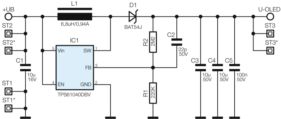
Bild 6: Schaltbild der Schaltreglerplatine PM2
