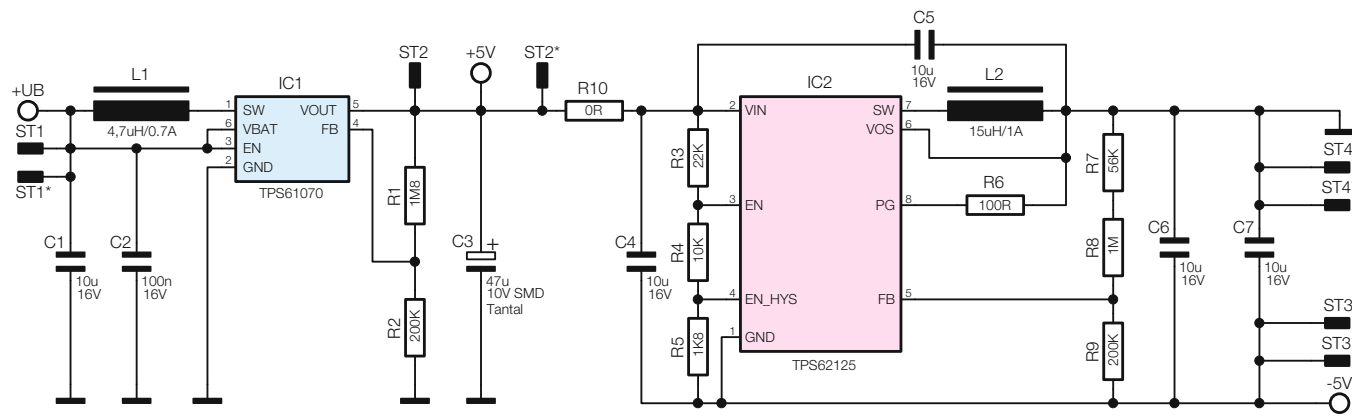
Bild 5: Schaltbild der Schaltreglerplatine PM1
