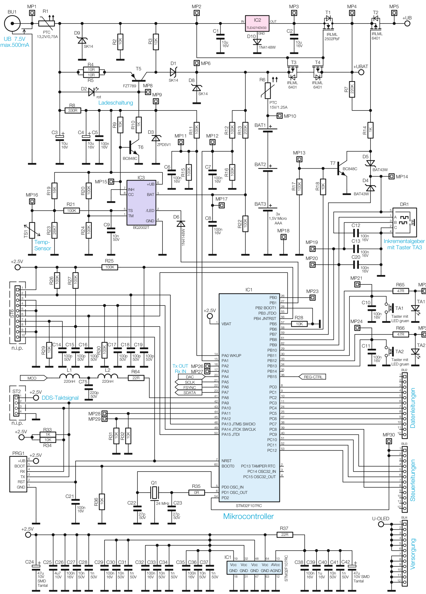
Bild 2: Schaltbild der Ladeschaltung und des Mikrocontrollerteils beim DDS101
