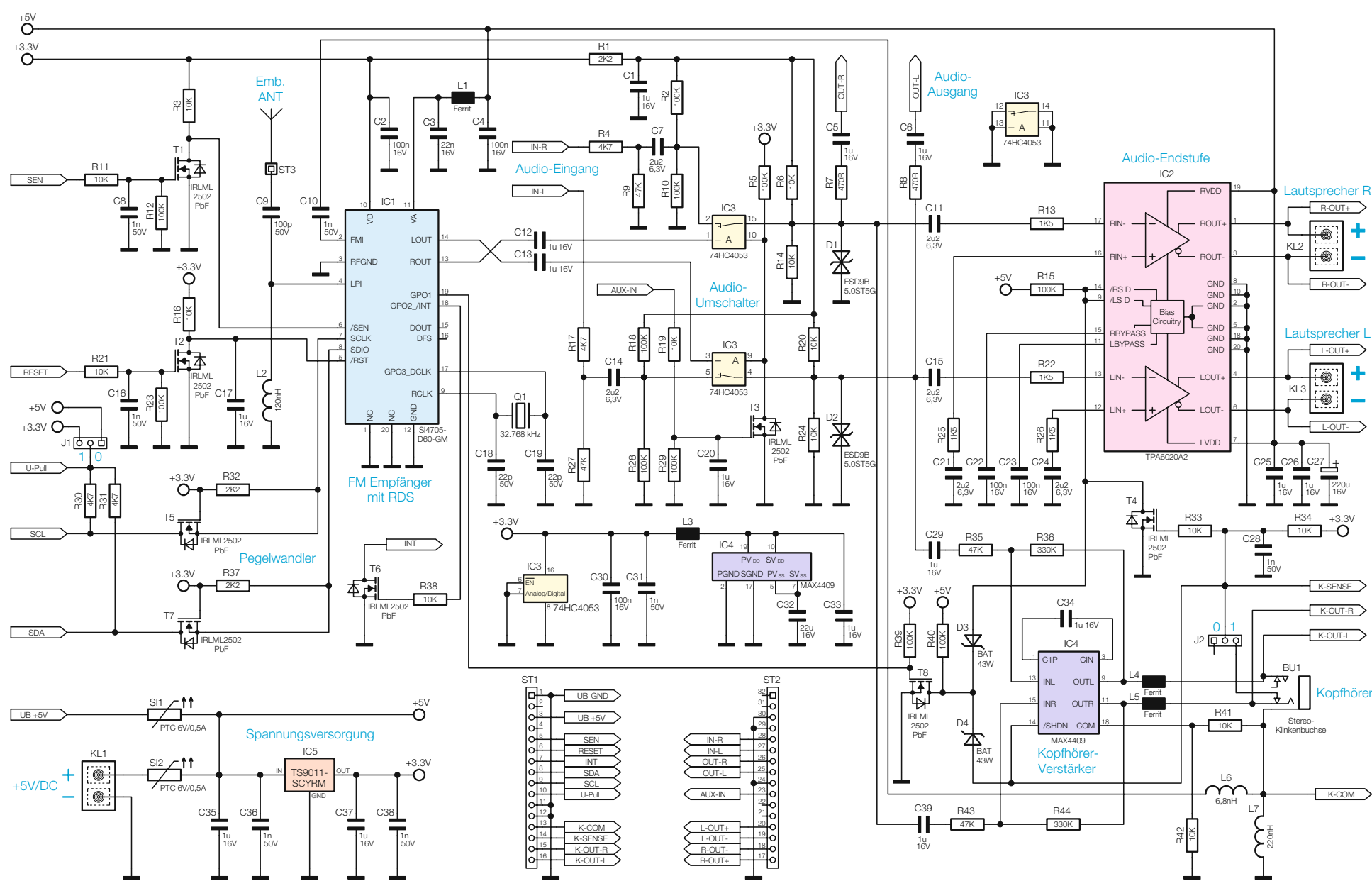
Bild 4: Das Schaltbild des kompletten Empfängers/Verstärkermoduls
