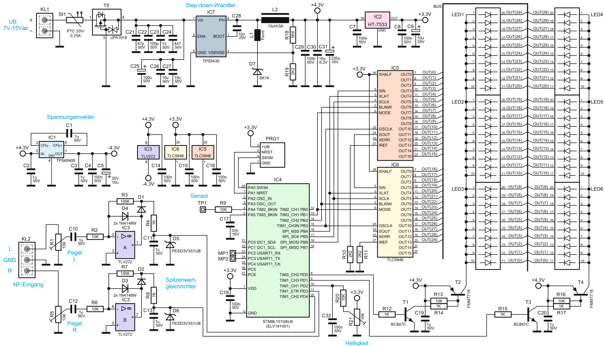
Bild 3: Das Schaltbild des VU-30
