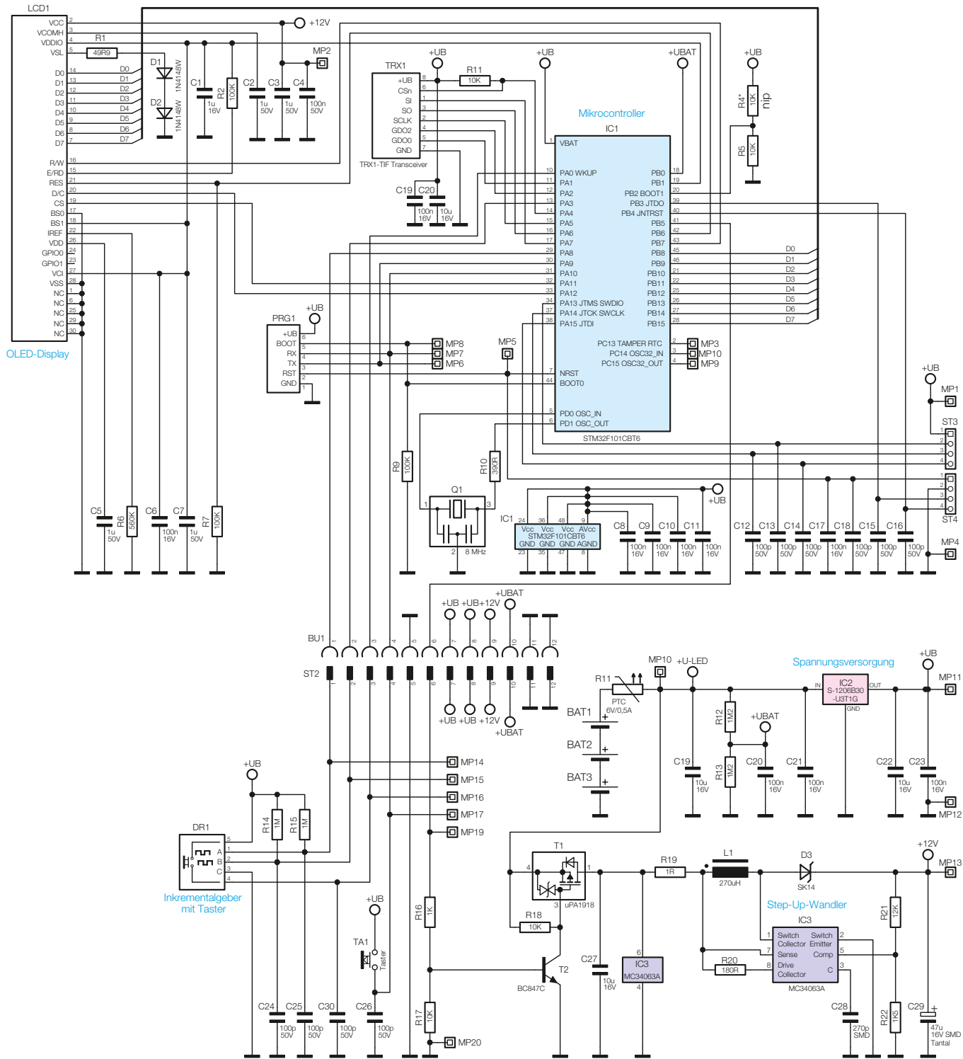
Bild 1: Schaltbild der Display-Fernbedienung
