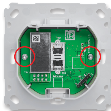
Bild 9: Die im Gehäuse verschraubte Control-lerplatine
