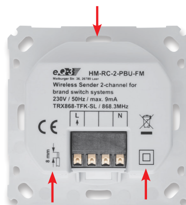
Bild 12: Das in die Montageplatte eingeklippte Gehäuse
