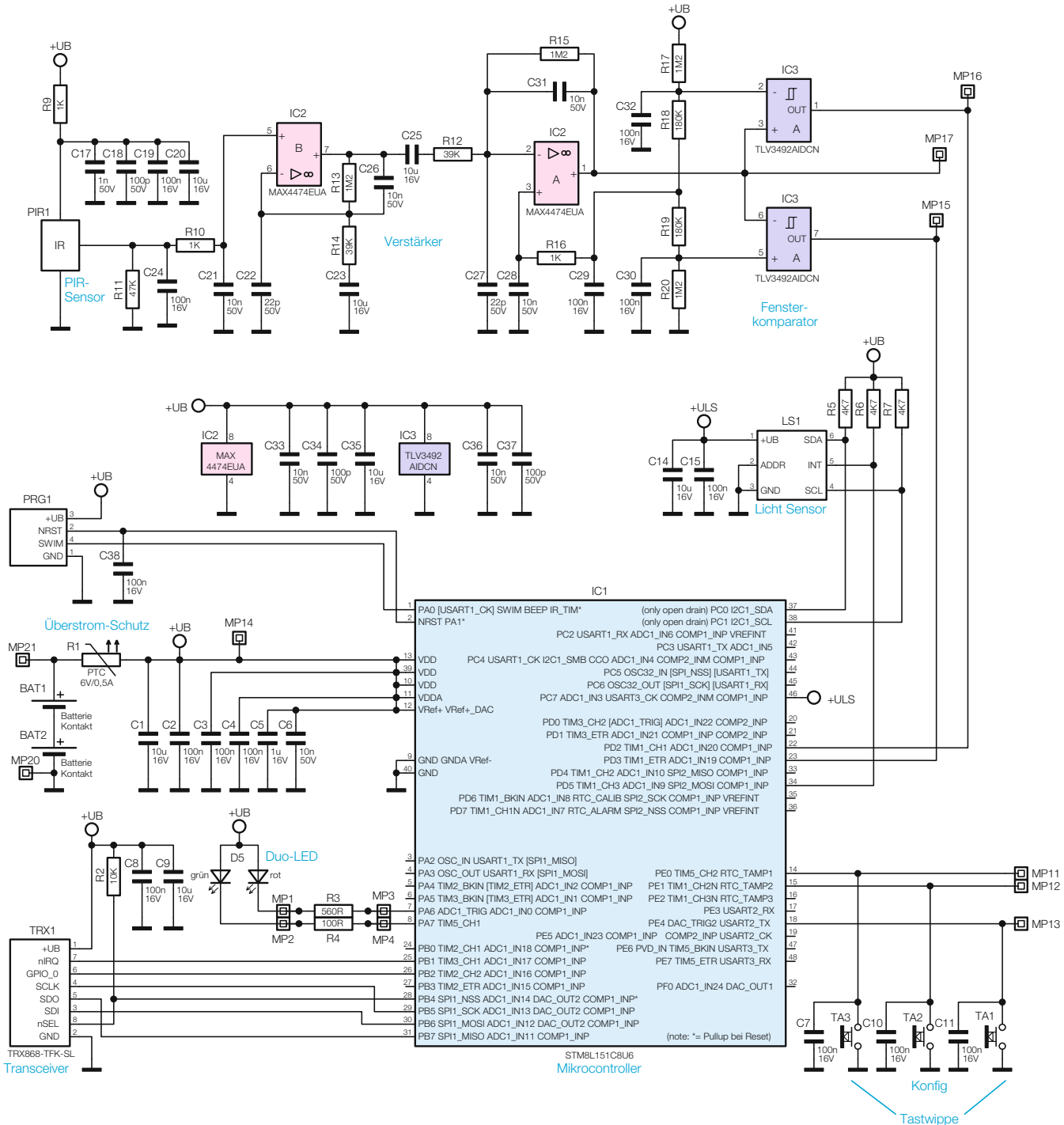
Bild 5: Das Schaltbild der Funk-Bewegungsmelder-Taster-Kombination
