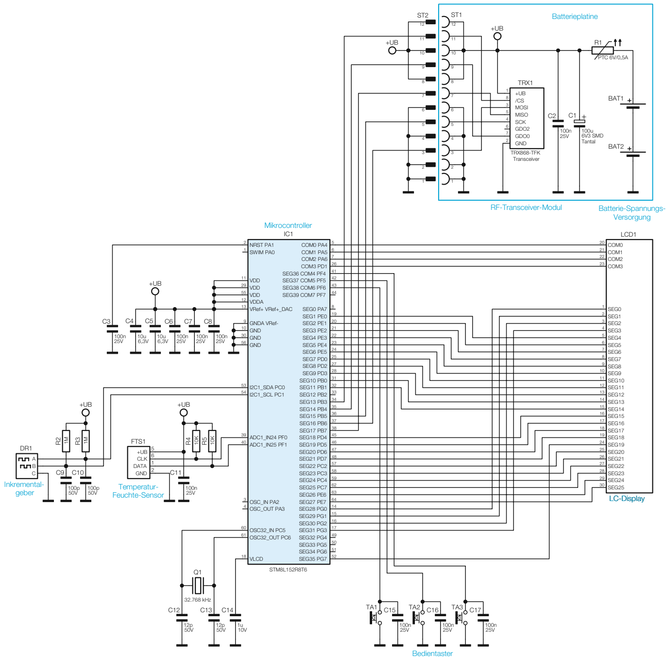
Bild 2: Schaltbild des HomeMatic-Wandthermostats
