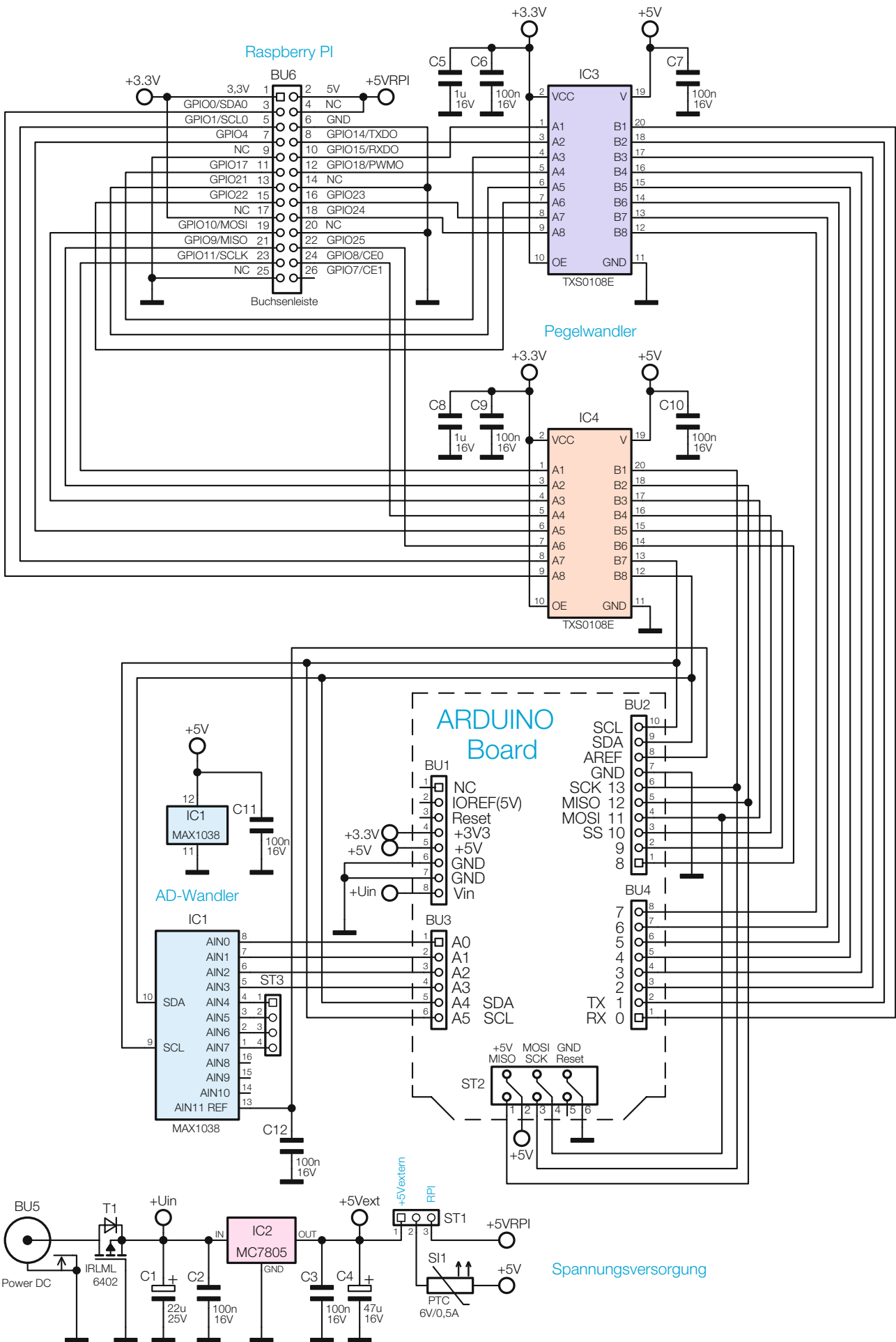
Bild 1: Das Schaltbild des Shield-Adapterboards RPi-AA1
