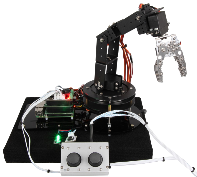
Abb. 1: Robot02 Inkl. optionalem Zubehör
