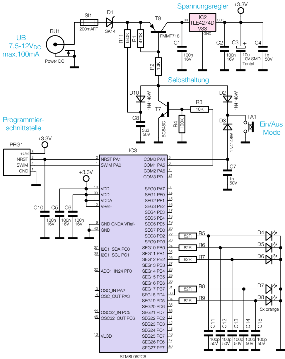
Bild 1: Schaltbild des Lichterbogens
