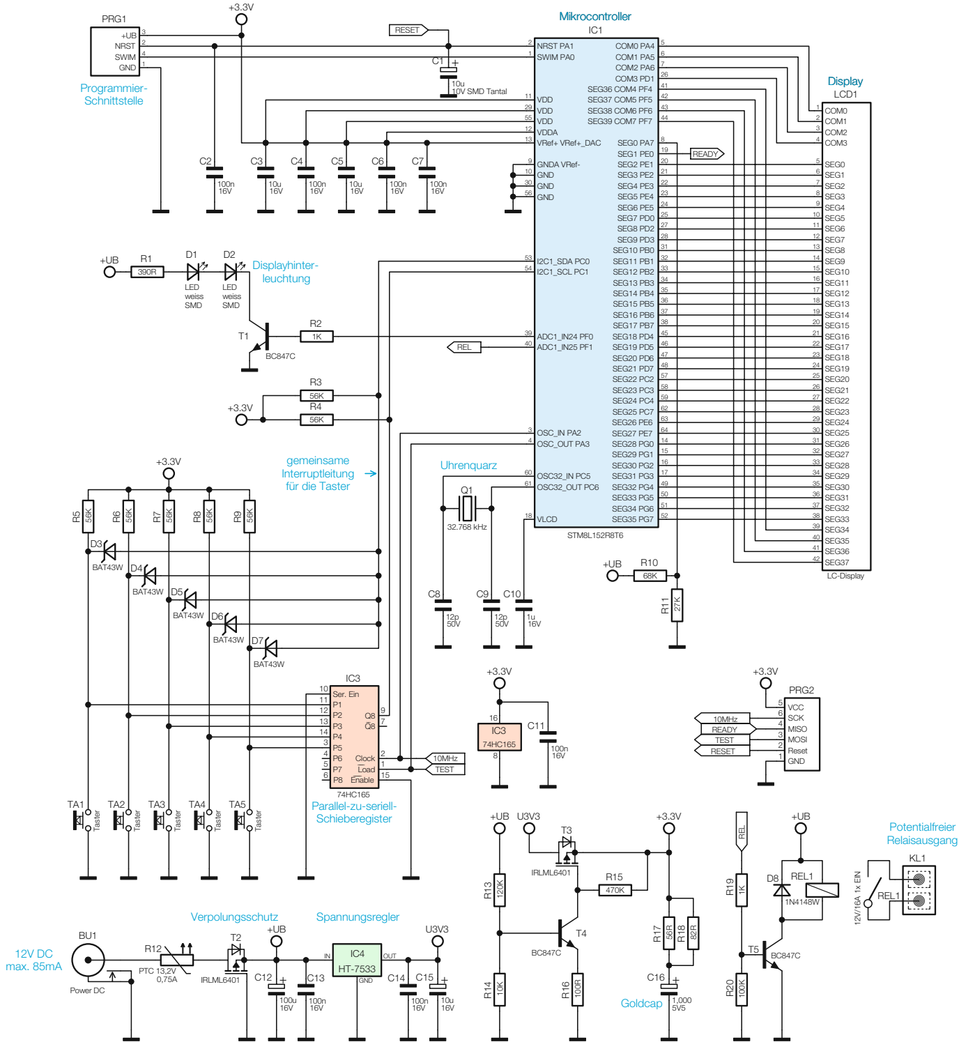
Bild 2: Das Schaltbild des Timermoduls WTMA1
