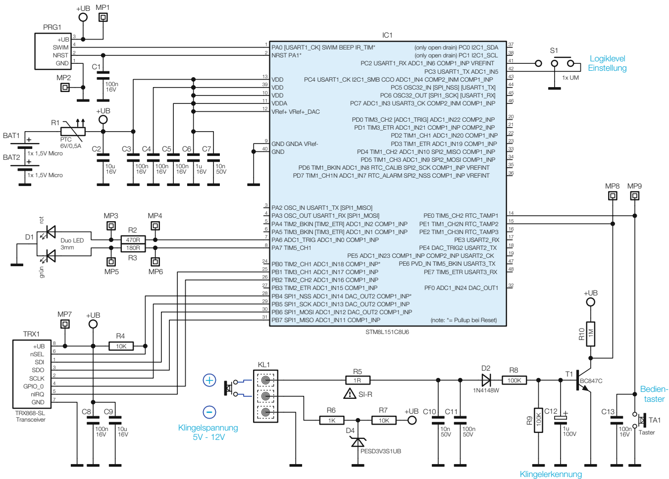
Bild 1: Das Schaltbild des Funk-Klingelsignalsensors
