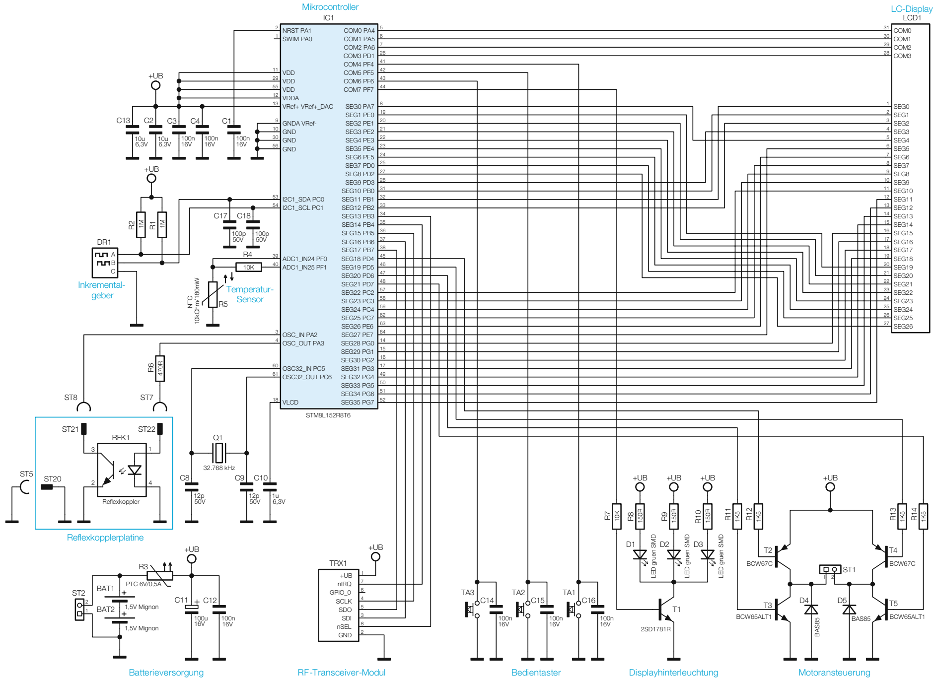
Bild 2: Das Schaltbild der Steuerungselektronik des Heizkörperthermostaten
