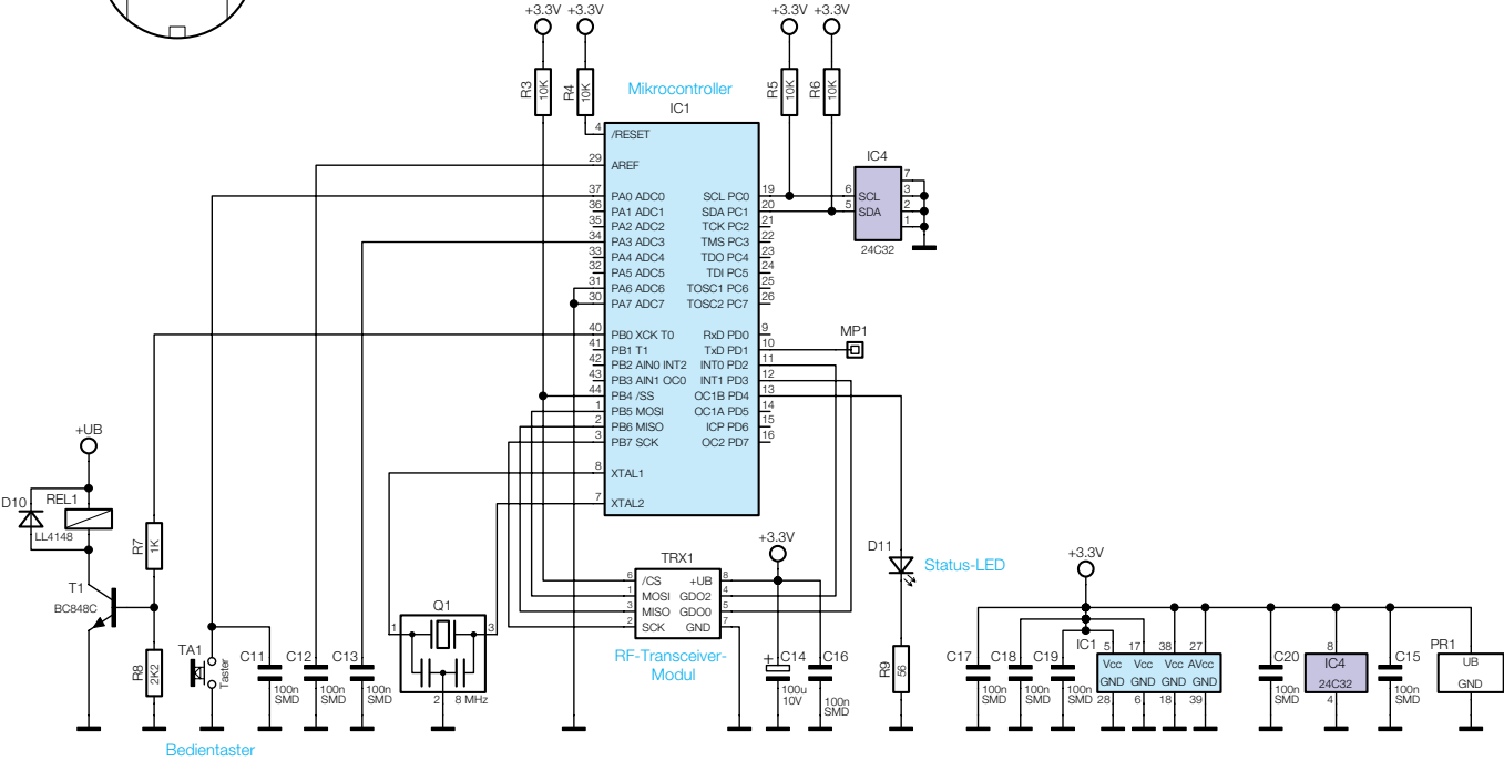
Bild 1: Schaltbild
