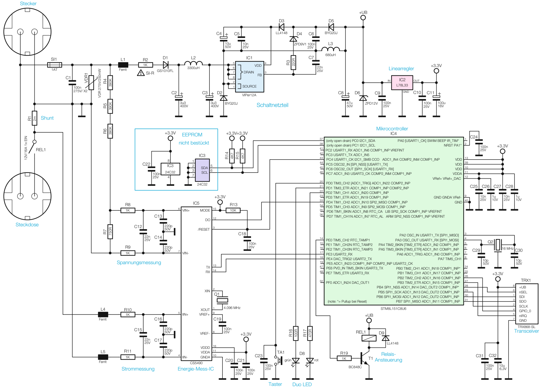
Bild 17: Das Schaltbild des HomeMatic-Funk-Schaltaktors mit Leistungsmessung
