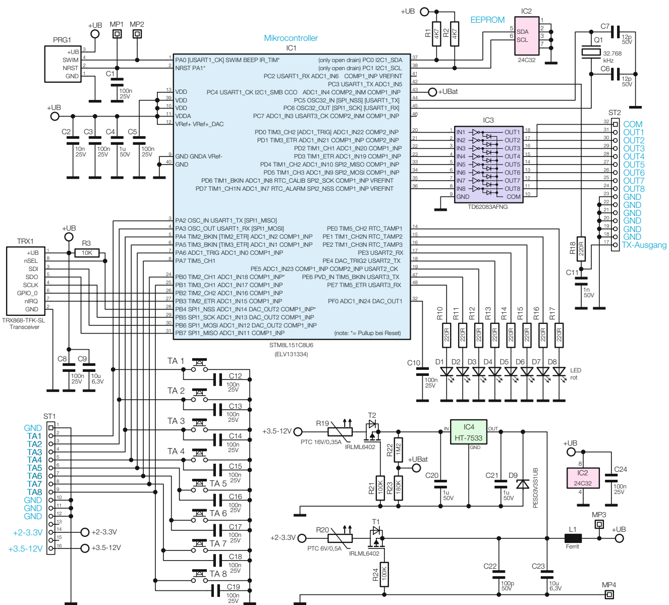
Bild 5: Das Schaltbild des 8-Kanal-Empfangsmoduls
