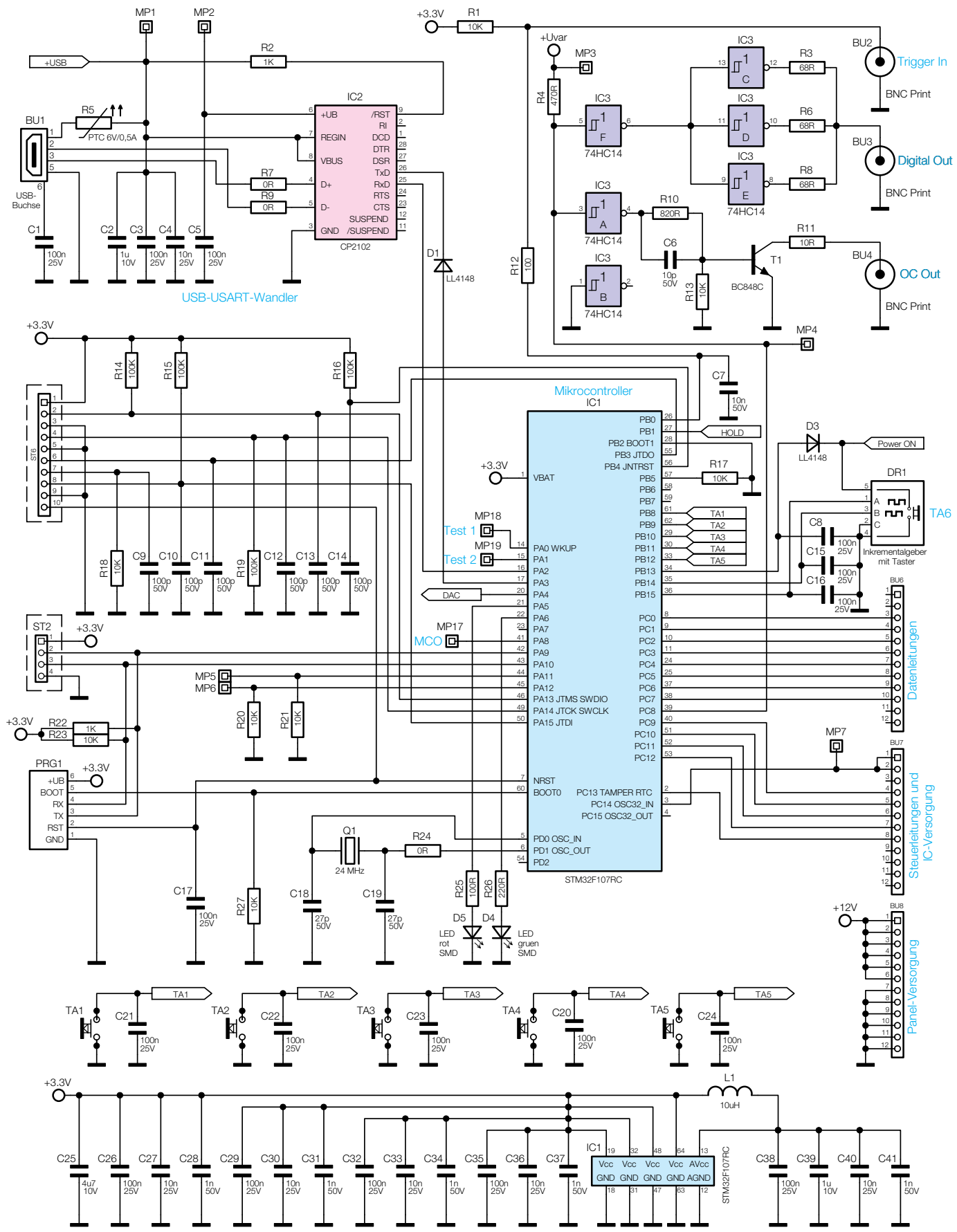
Bild 2: Schaltbild des Mikrocontrollers mit angeschlossener Peripherie
