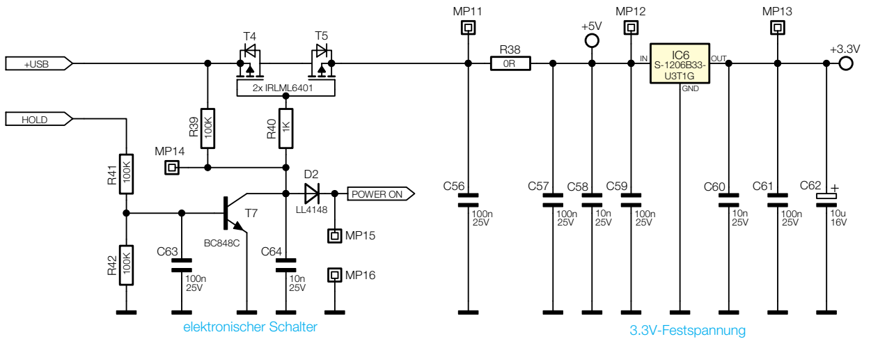
Bild 1: Schaltbild der einzelnen Spannungsversorgungen
