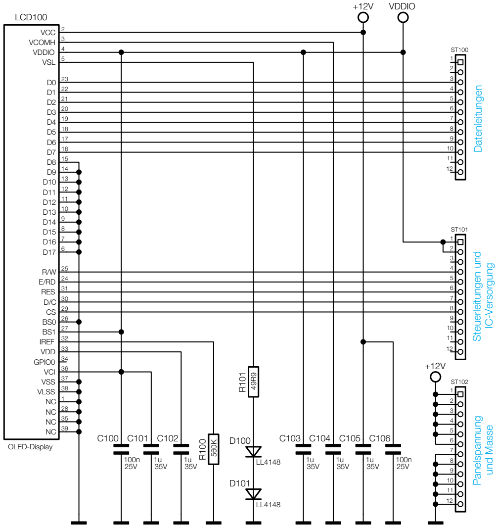
Bild 3: Schaltbild des OLED-Displays
