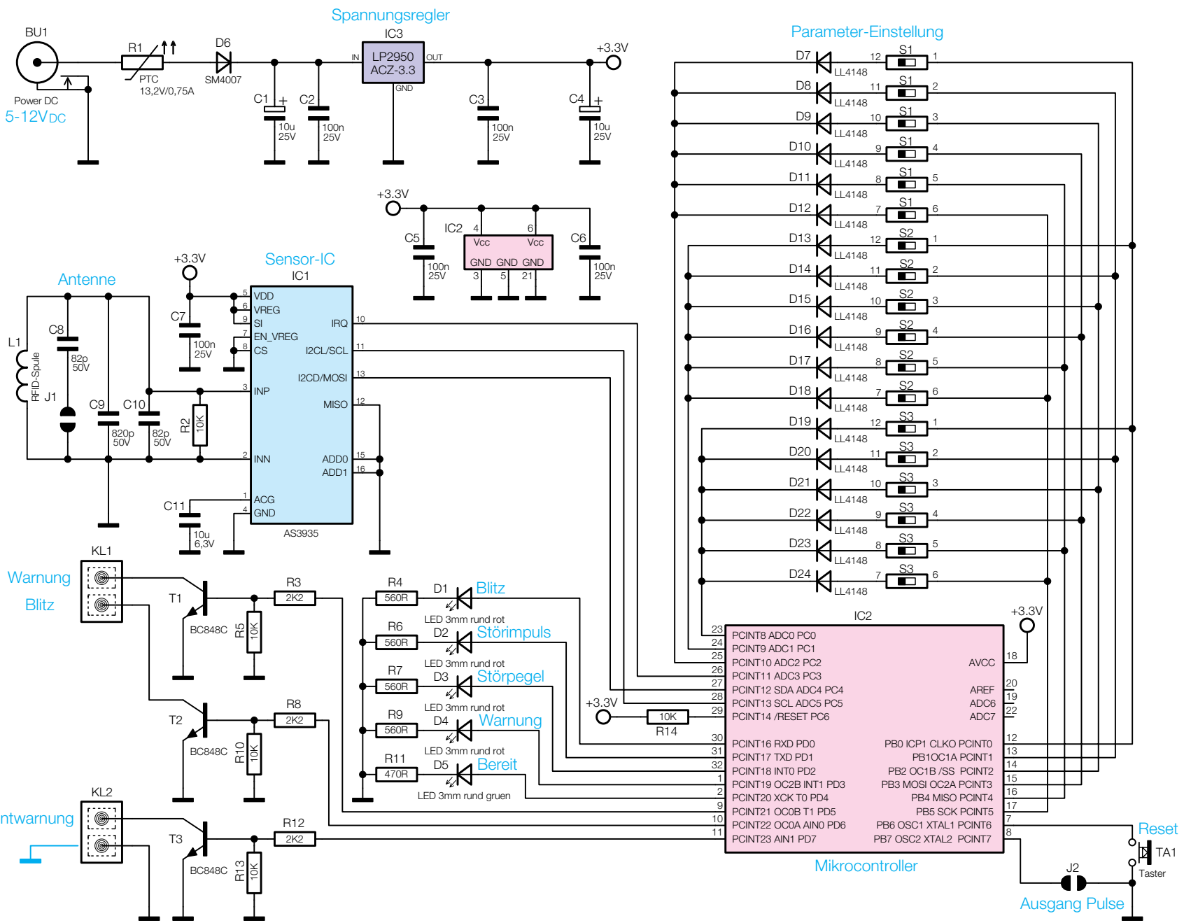
Bild 1: Schaltbild des Gewitterwarners
