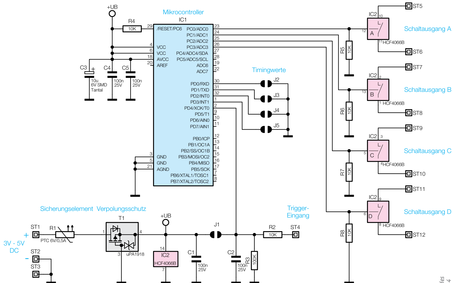
Bild 3: Das Schaltbild des Einschaltautomaten EA4
