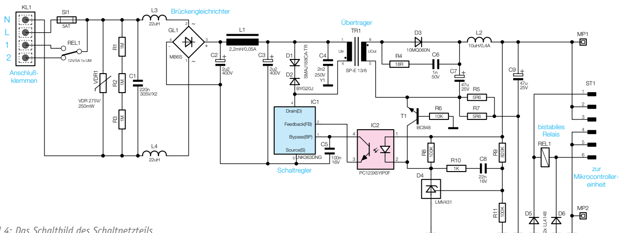
Bild 4: Das Schaltbild des Schaltnetzteils
