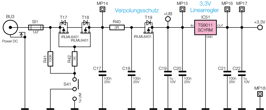
Bild 7: Das Schaltbild der Spannungsversorgung des MSB1
