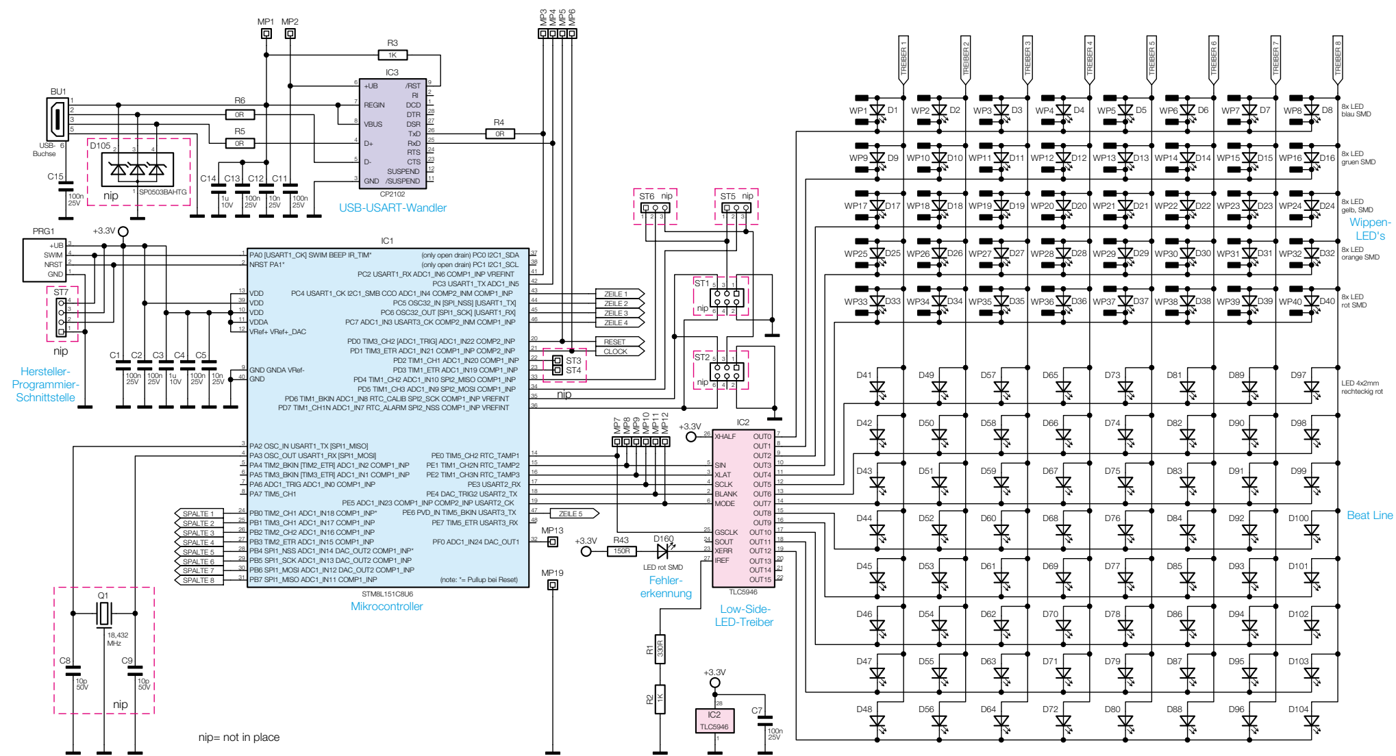
Bild 8: Die Schaltung des Mikrokontrollerteils mit angeschlossener Peripherie und LED-Matrix
