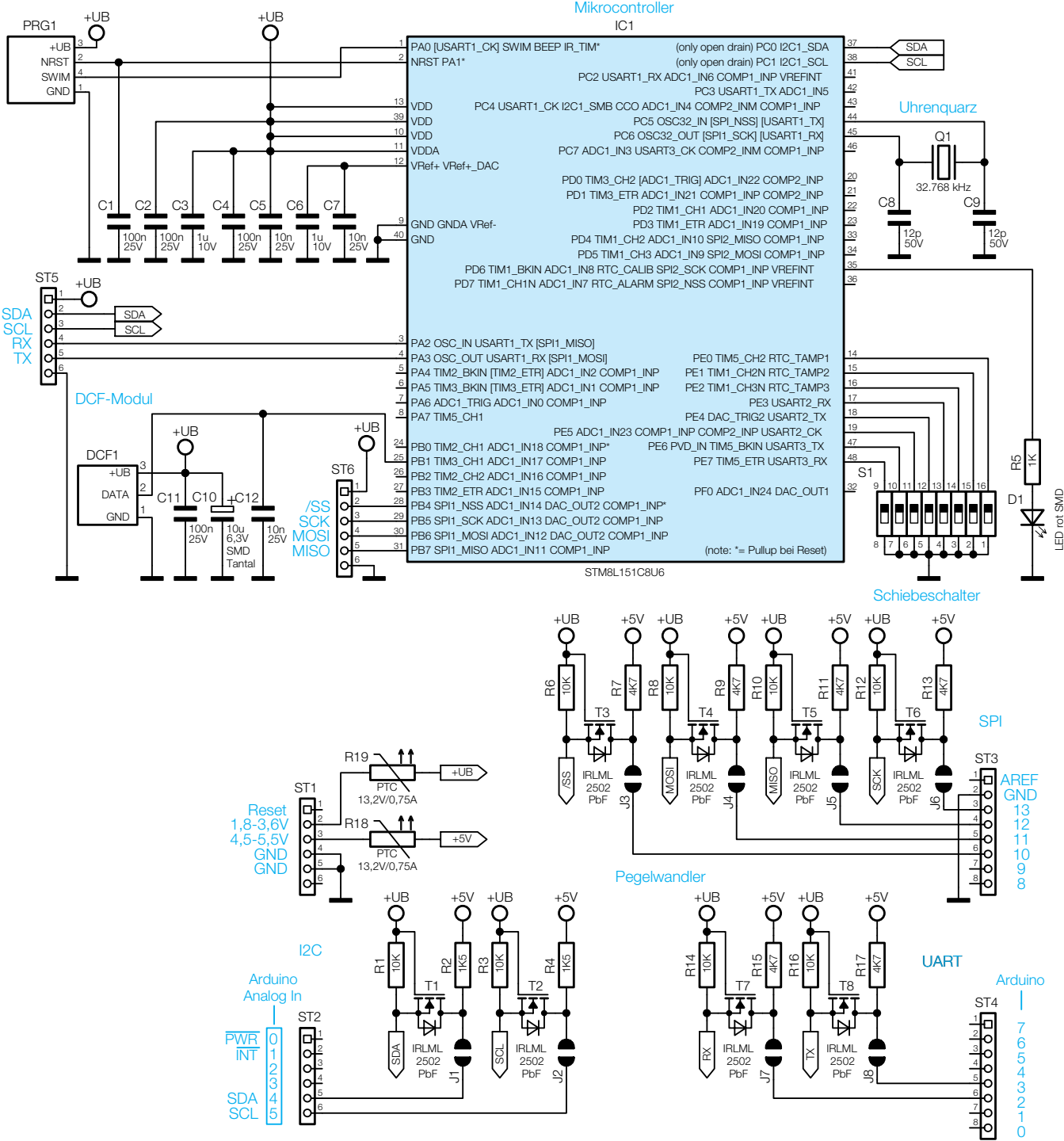
Bild 1: Schaltbild des RTC-DCF-Moduls
