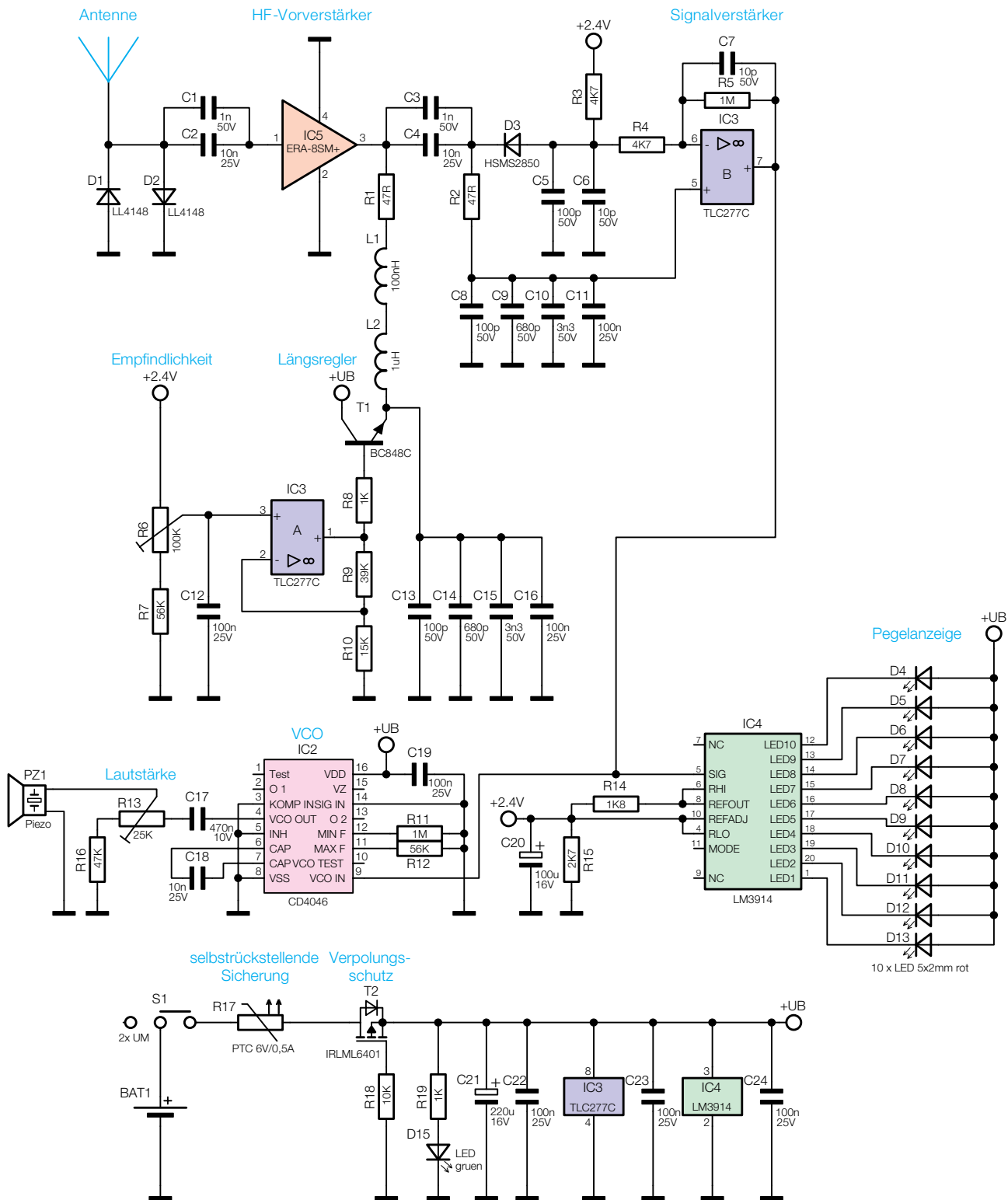
Bild 2: Das Schaltbild des Wanzenfinders WF 2
