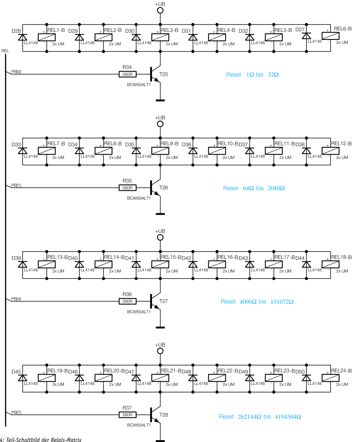
Bild 4: Teil-Schaltbild der Relais-Matrix
