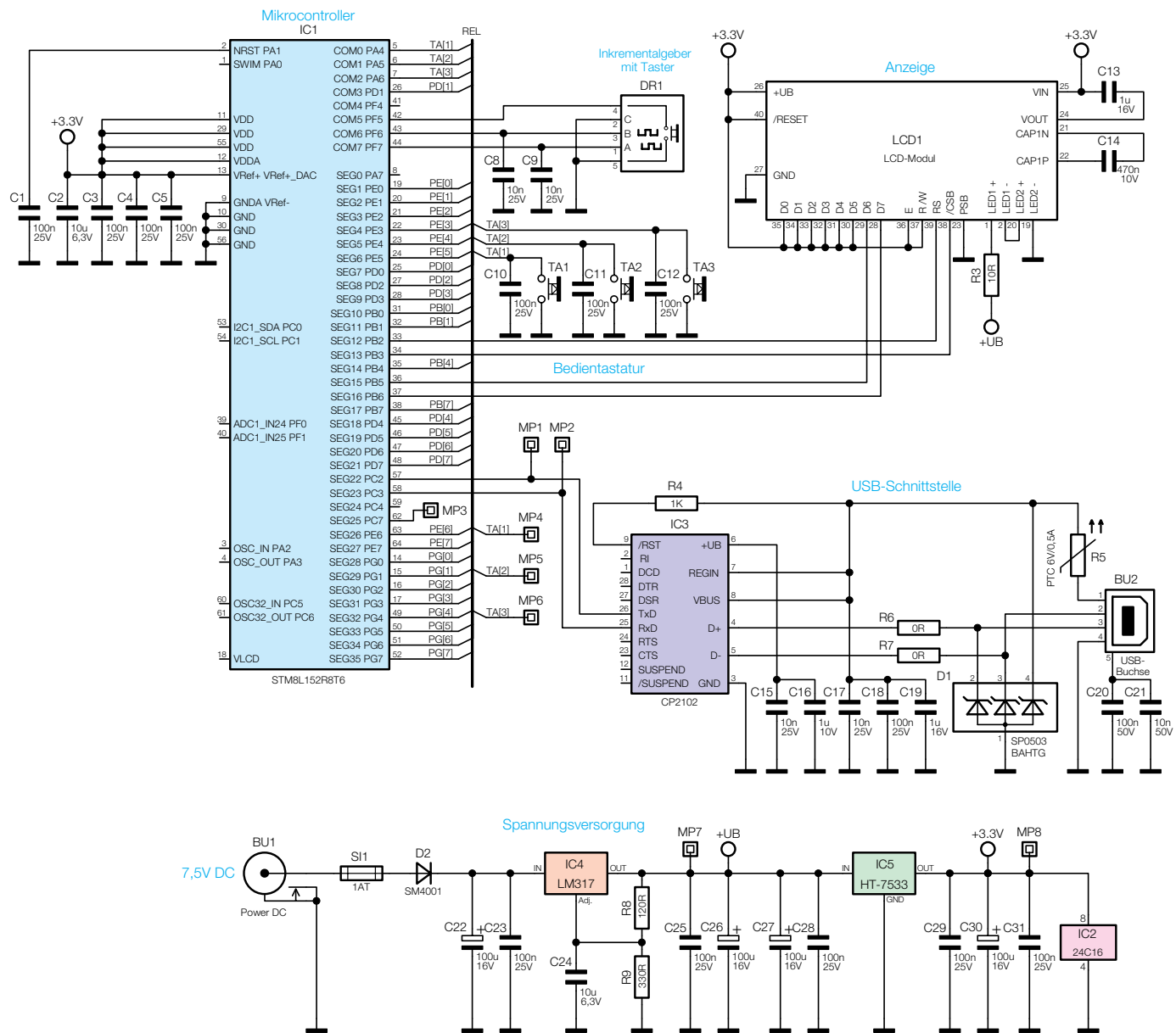
Bild 2: Das Schaltbild der Steuerung der EWD 100
