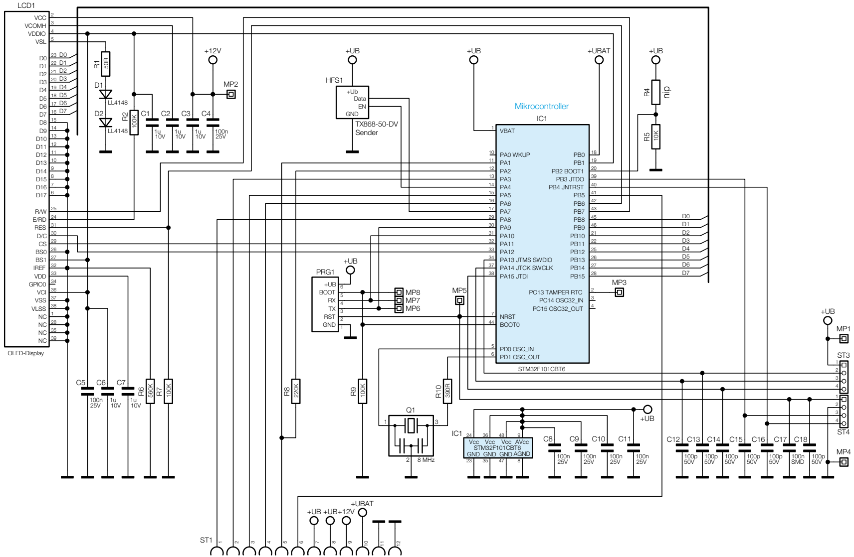
Bild 4: Das Schaltbild der Displayplatine
