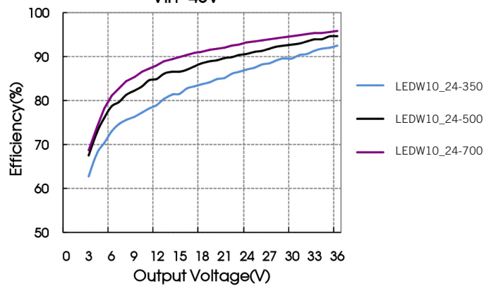
Vin=48V
