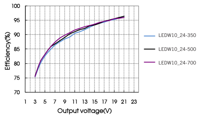
Vin=48V
