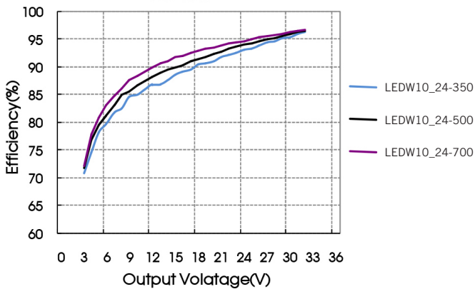
Vin=36V
