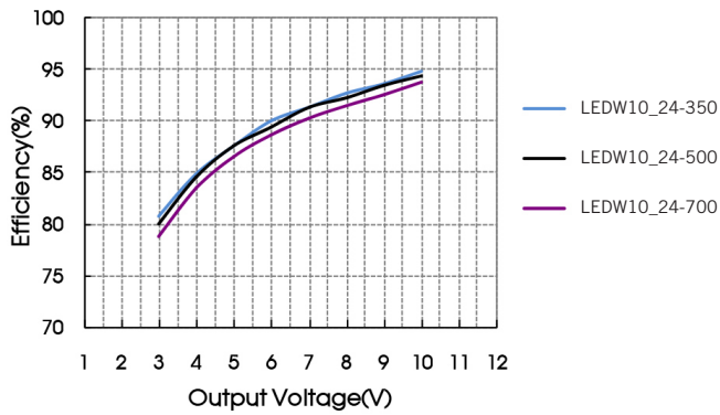
Vin=36V
