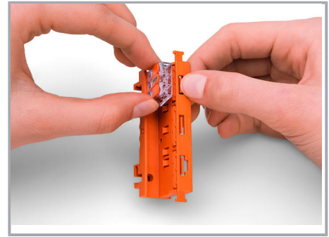
Lösen der Verbindungsklemme aus dem Befestigungsadapter
