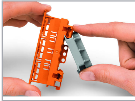
Verrasten des Universalwinkeladapters (222-510) an den Befestigungsadapter
