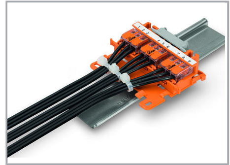
Liegende Montage auf Tragschiene 35 mittels Universalwinkeladapter
