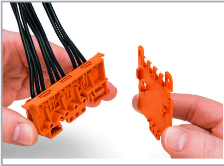
Montage der Zugentlastungsplatte (222-505) an den Befestigungsadapter
