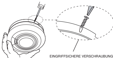
gewindeschneidende Schraube
