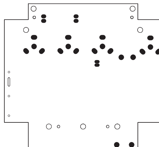
BOTTOM MASK
