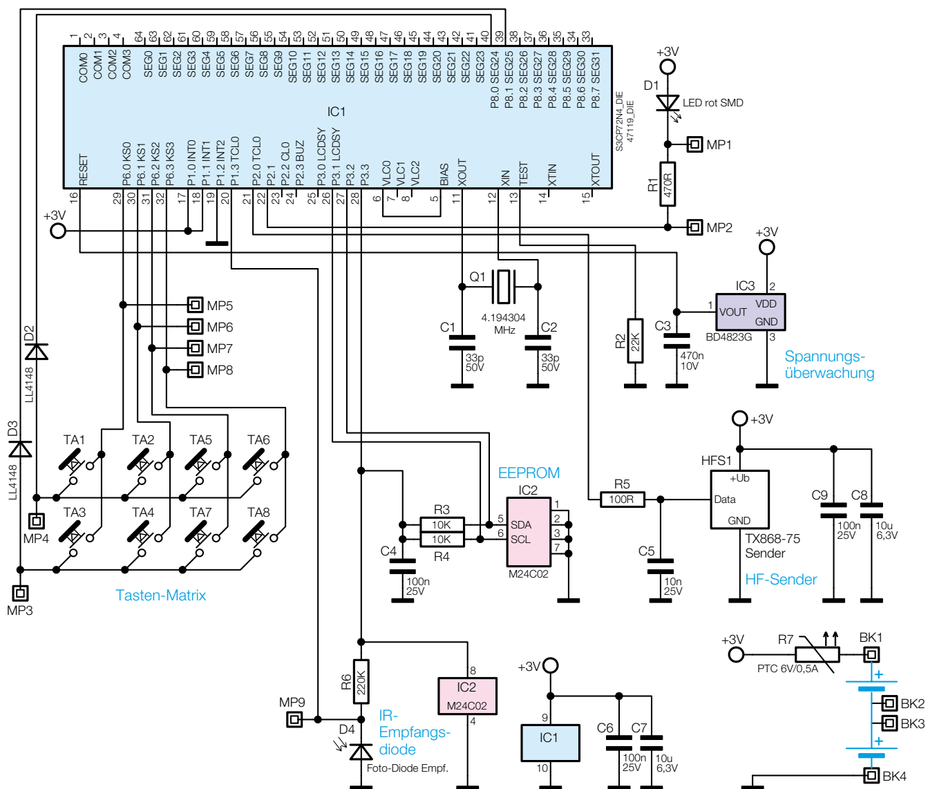
Bild 1: Das Schaltbild der FS20 S8-3
