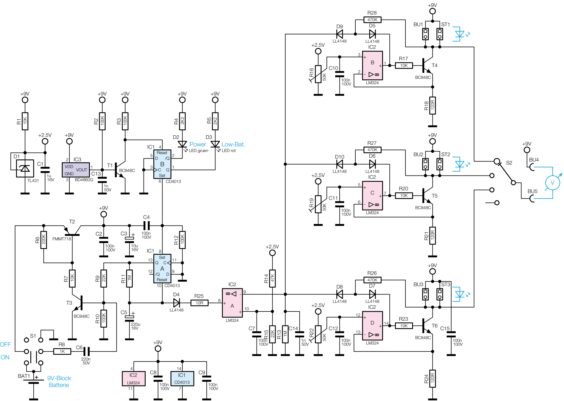
Bild 1: Das Schaltbild des LED-Testers
