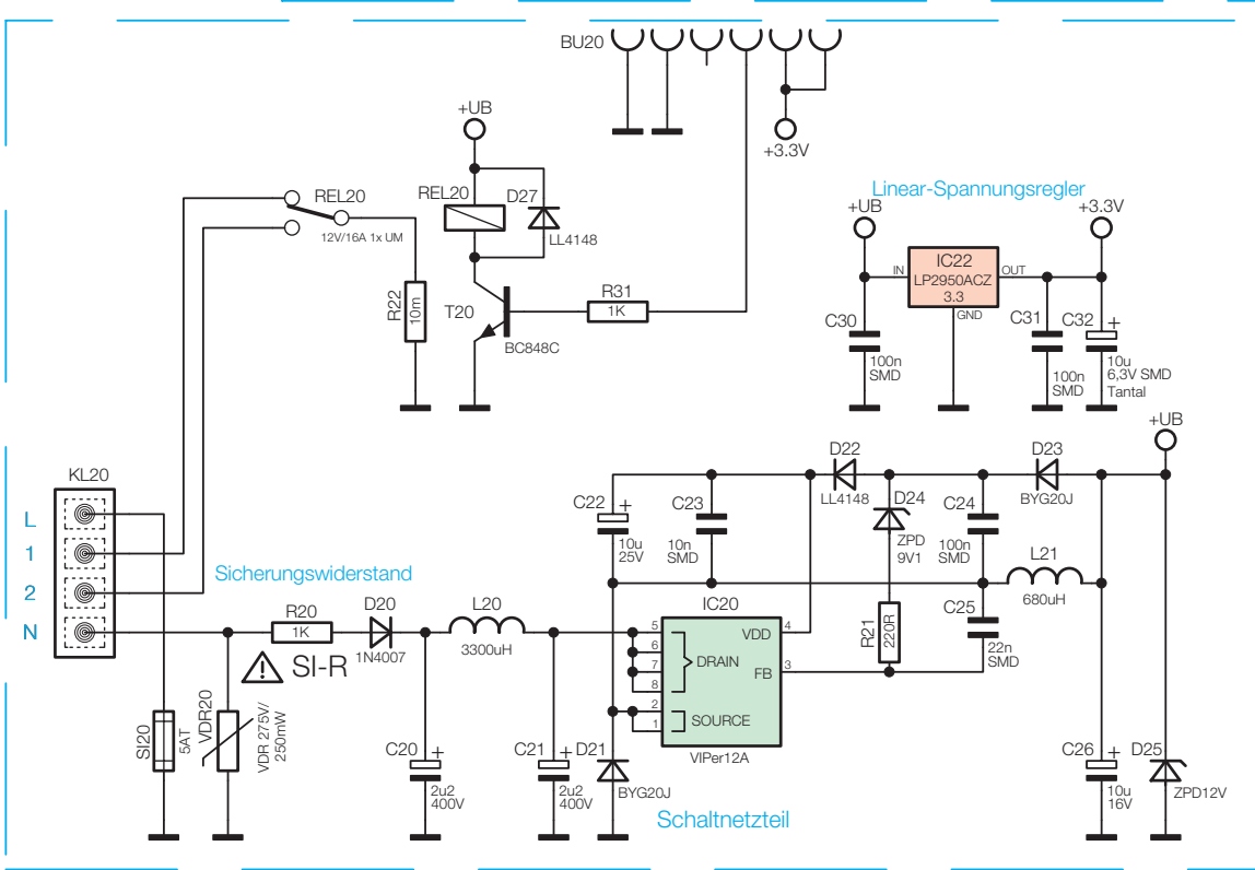
Bild 1: Schaltbild des ST55UP, oben der Controller-, unten der Leistungsteil
