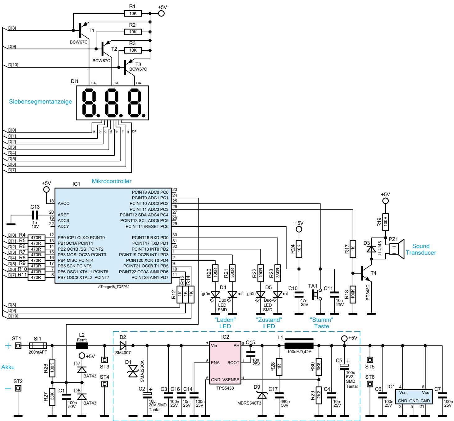
Bild 1: Das Schaltbild des BW100
