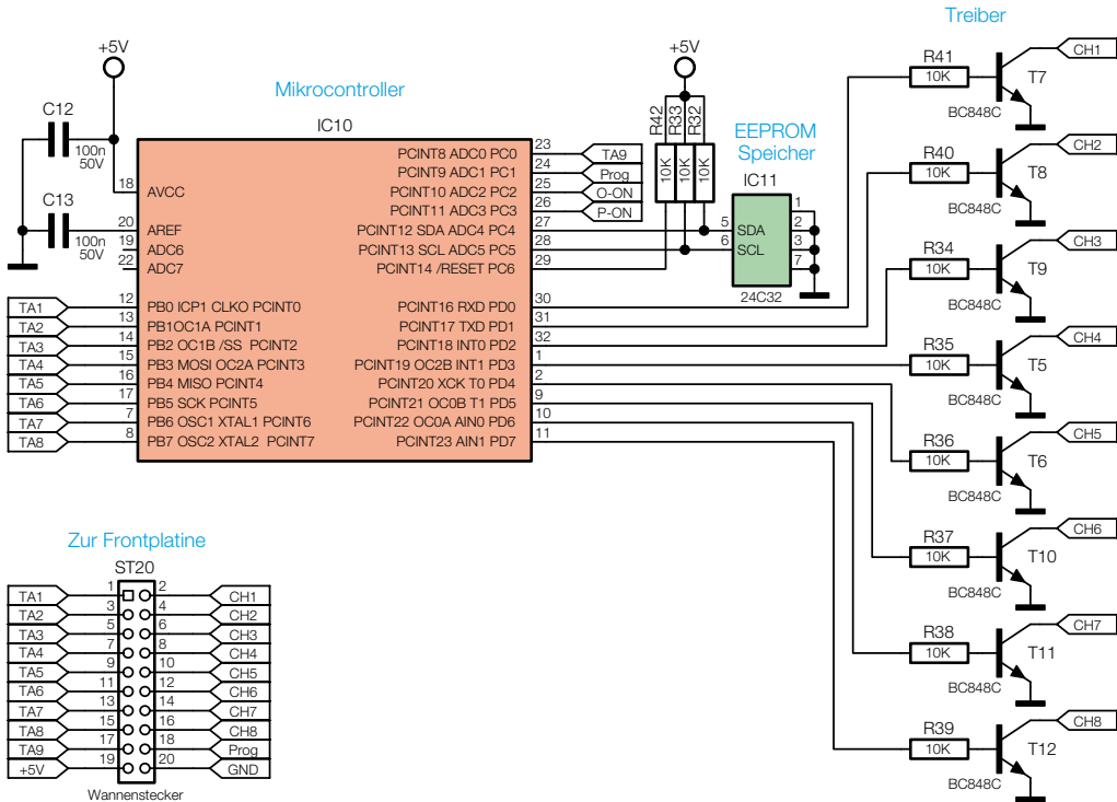
Bild 2: Das Schaltbild des Digitalteils mit Prozessor, EEPROM und Optokoppler-Ansteuerung
