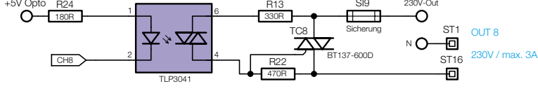
Bild 3: Das Schaltbild des Leistungsteils
