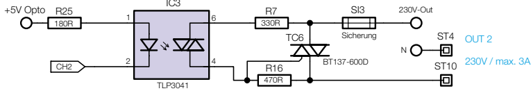
Ansteuerung OUT 3
