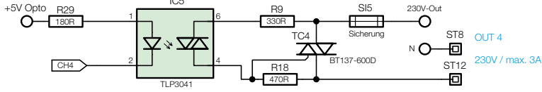
Ansteuerung OUT 5
