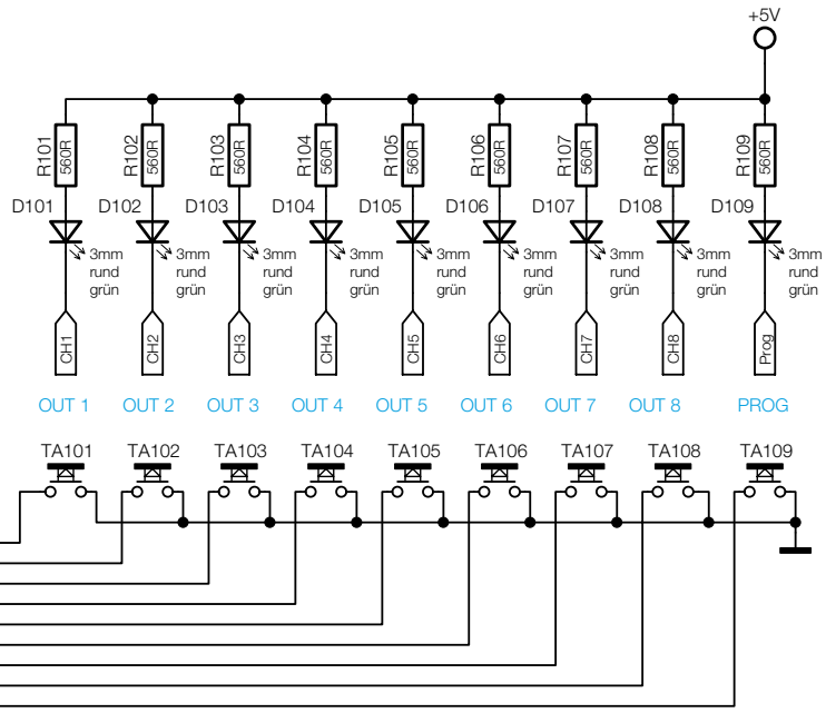
zur Basisplatte
