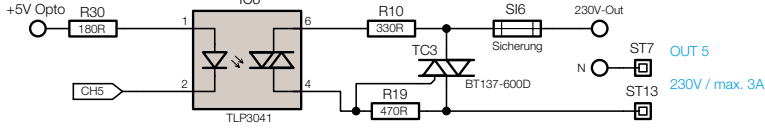
Ansteuerung OUT 6
