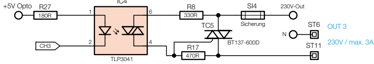
Ansteuerung OUT 4
