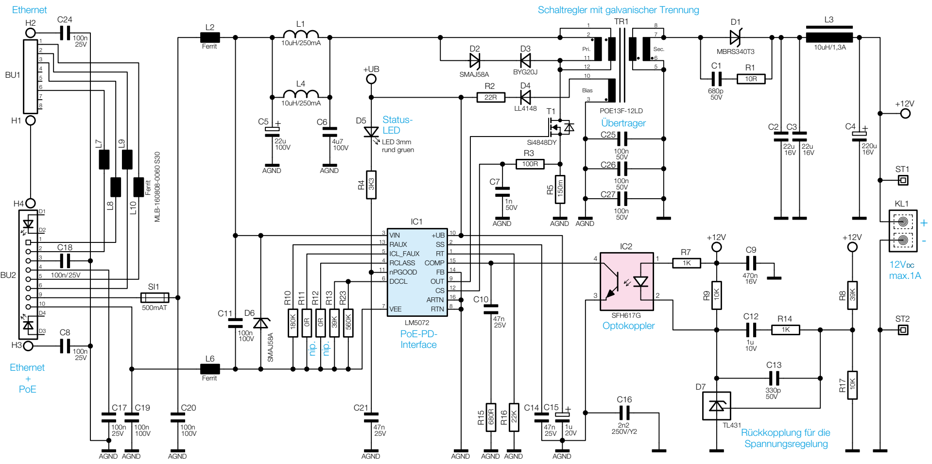
Bild 3: Die Schaltung des PoE-S mit dem PD-Interface-Baustein LM5072 als zentralem Bauelement
