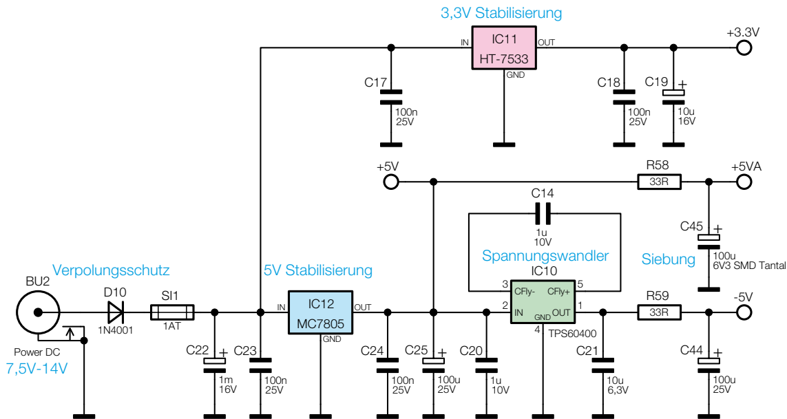
Bild 7: Spannungsversorgung des MD0100
