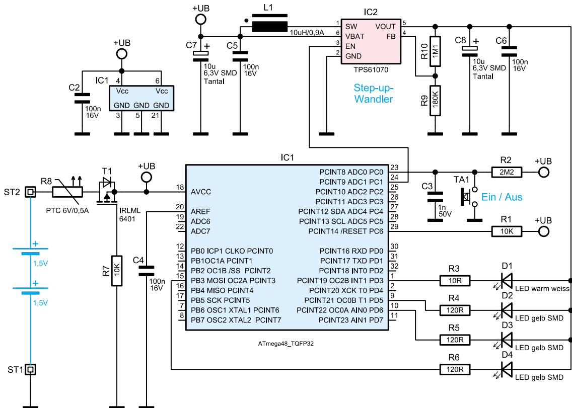
Bild 4: Die Schaltung der LED-Flackerkerze
