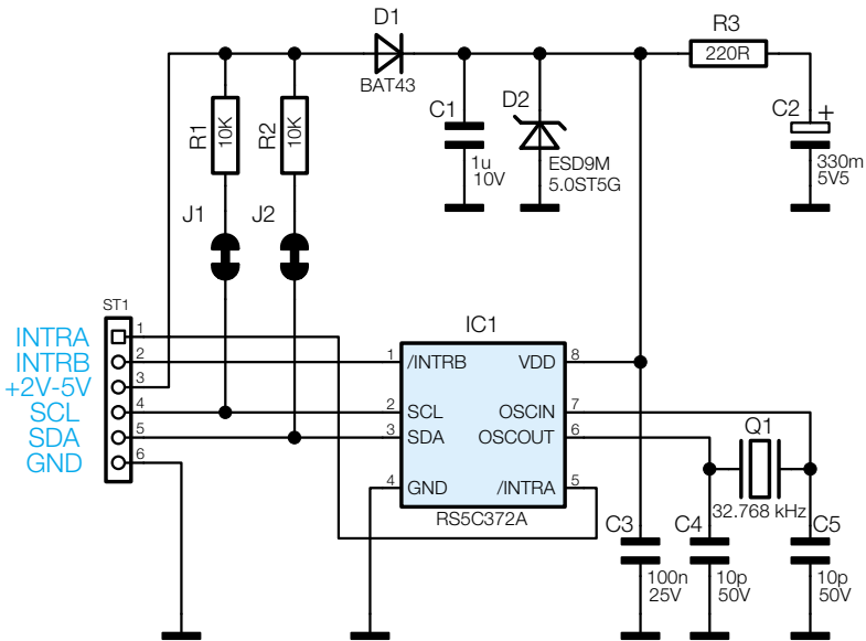
Bild 2: Das Schaltbild des I 2 C-RTC
