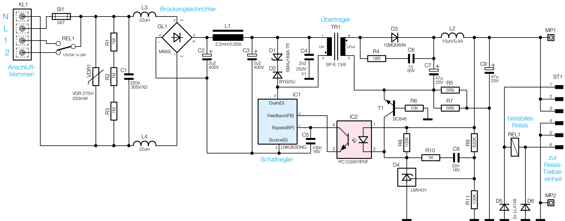
Bild 4: Schaltnetzteil des UTH100 UP
