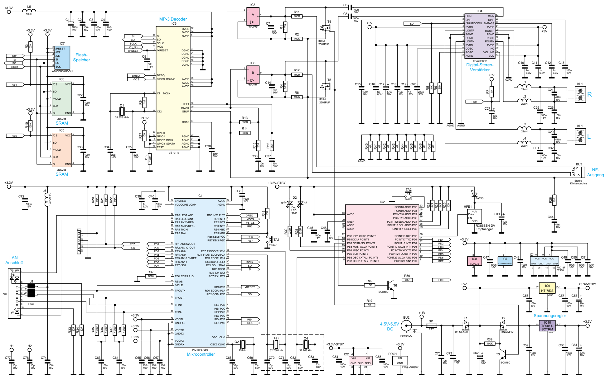
Bild 14: Schaltplan des FS20 IRB
