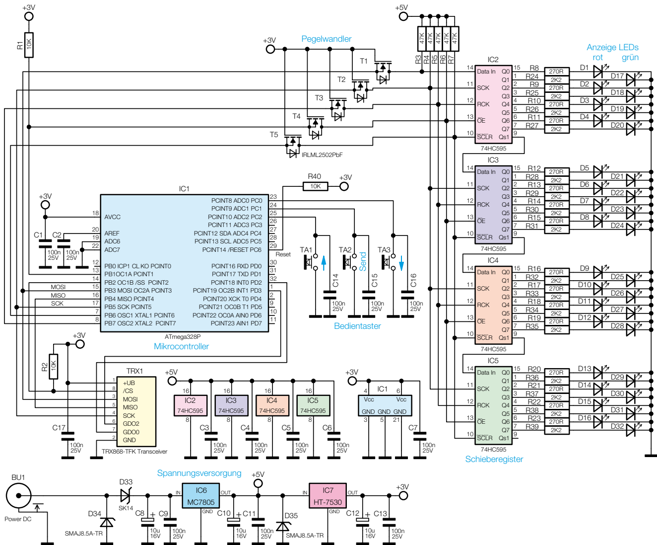
Bild 3: Das Schaltbild der HomeMatic-Statusanzeige
