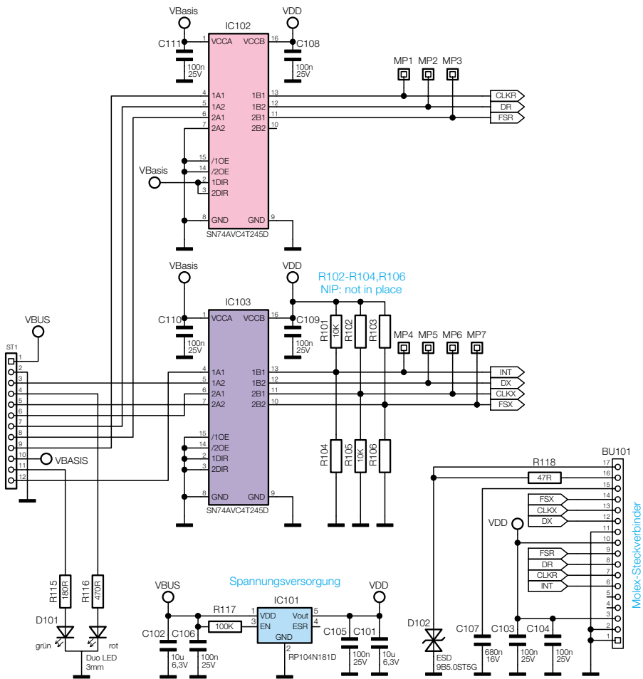
Bild 2: Die Sensor-Schaltung
