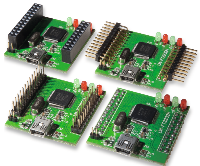
Bild 7: Verschiedene Bestückungsvarianten mit Buchsen und Stiftleisten. Die Standardversion befindet sich vorne links.
